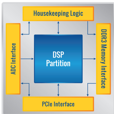
ATS9373 FPGA
